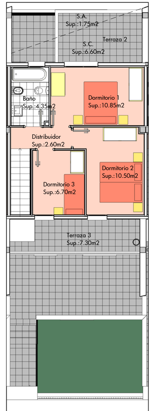
Planta Primera
